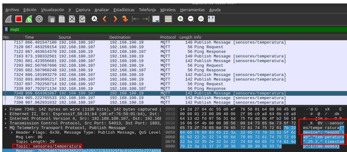
Figura 2.3: Lecturas de telemetría visible en paquete PUBLISH. El JSON es completamente legible por cualquier sniffer en la red.
