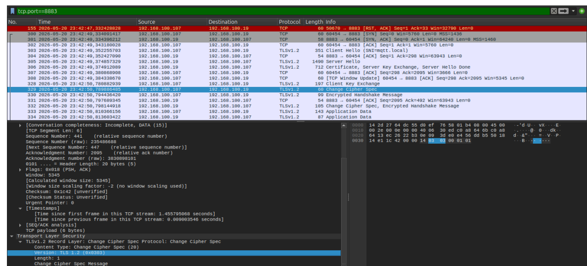
Figura 3.3: Cambio de especificación de cifrado (Change Cipher Spec) y establecimiento final de la capa segura. El canal ahora se encuentra cifrado.
