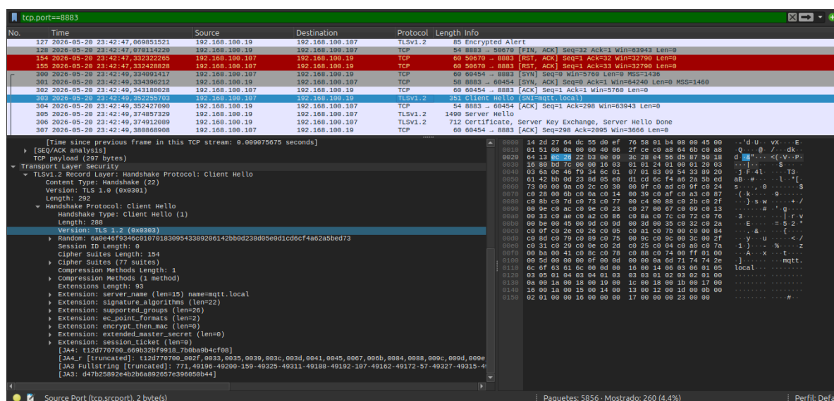
Figura 3.1: Trama Client Hello. El ESP32 inicia la negociación TLS proponiendo las suites criptográficas disponibles.
