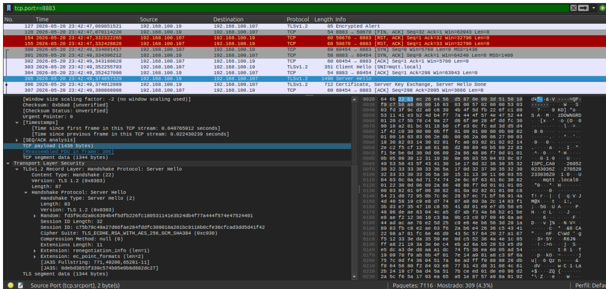
Figura 3.2: Tramas Server Hello, Certificate y Server Key Exchange. El broker elige los parámetros criptográficos y transmite su certificado server.crt firmado por la CA del ISPC.
